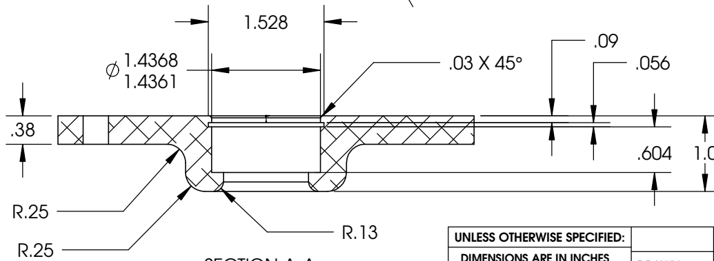
SECTION A-A SCALE 1 : 1.75
